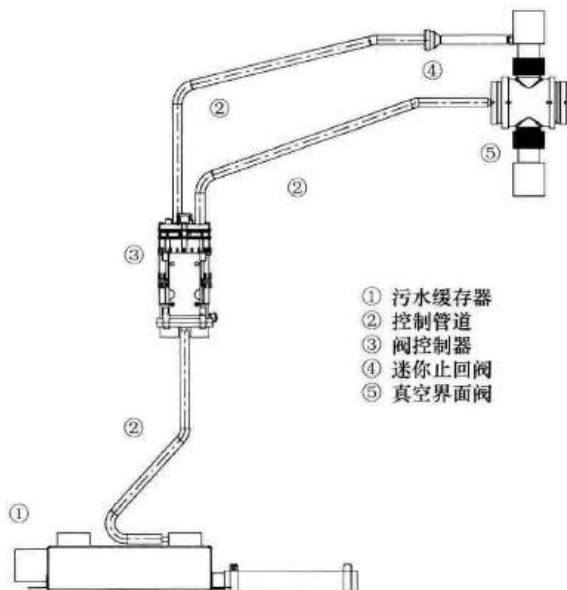
图5 真空界面单元（地漏、真空界面阀单元、 冷凝水收集装置）原理示意
