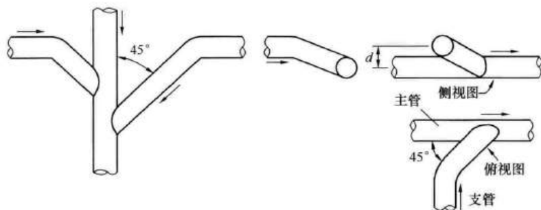
图 16 支管铺设基本原则
