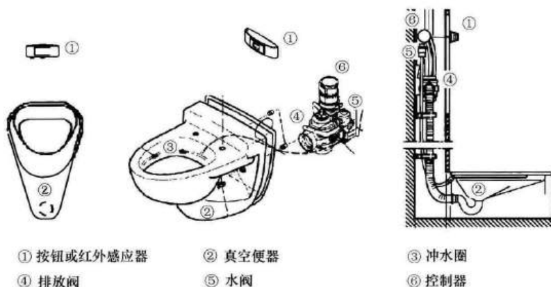
图 4 真空坐（蹲）便器组成示意
