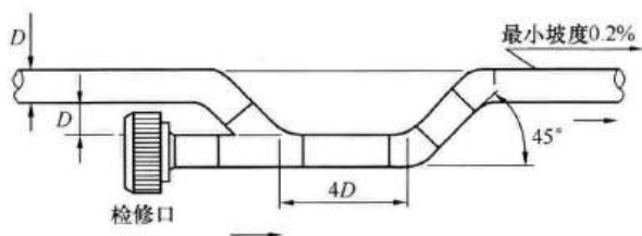
图 14 输送集水弯标准尺寸示意
