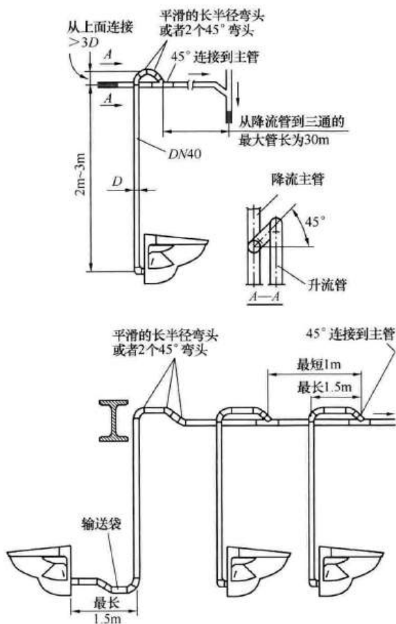
图 17 真空界面单元提升管设置的基本原则
