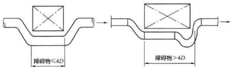
图 15 障碍物处输送集体弯的铺设方法
