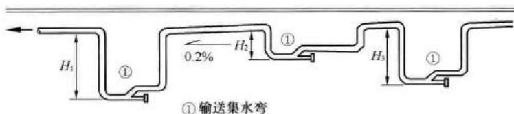
图9 真空排水管道 U形输送集水弯铺设方式示意
