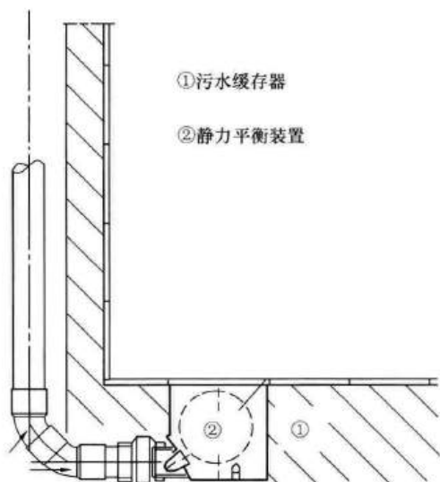
图6 真空吸水器原理示意
