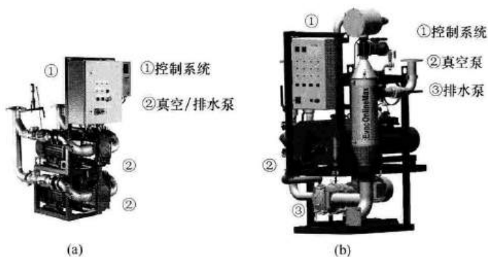
图 8 无真空罐的真空泵站组成示意
