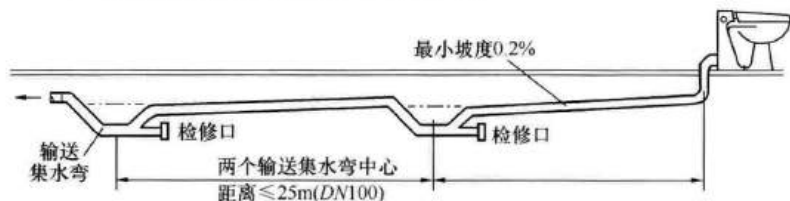
图 13 DN100 理想管道铺设示例
