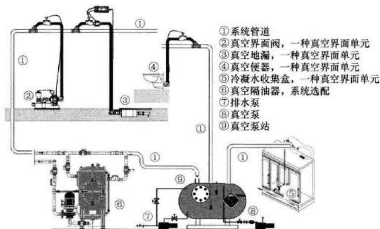
图1 真空排水系统组成示意
