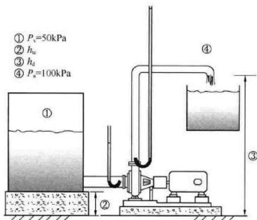
图 10 扬程计算示意
