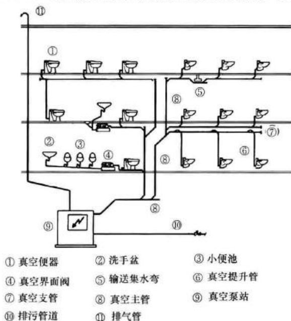
图 2 真空管道及附件组成示意
