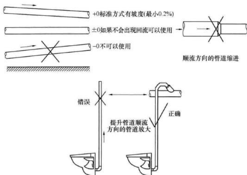
图 18 严格禁止的管道铺设方式
