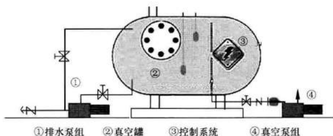
图7 配备真空罐的真空泵站组成示意
