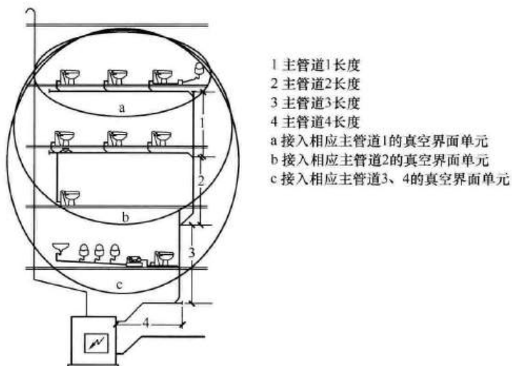
图 11 管道分段计算模型示意
